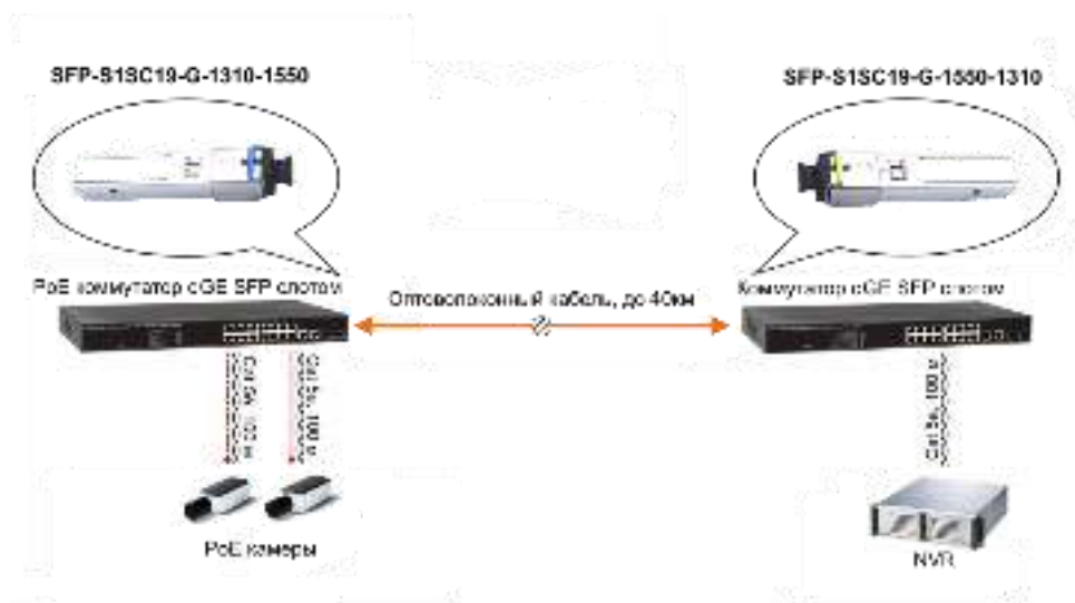
Рис.6 Типовая схема подключения SFP модулей SFP-S1SC19-G-1310-1550, SFP-S1SC19-G-1550-1310
