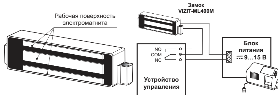
Рисунок 4 - Рабочая поверхность электромагнита
