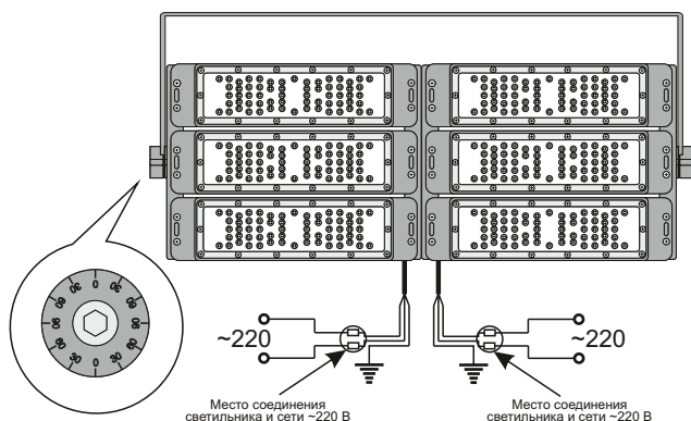
Рисунок 2 — Схема подключения изделия
