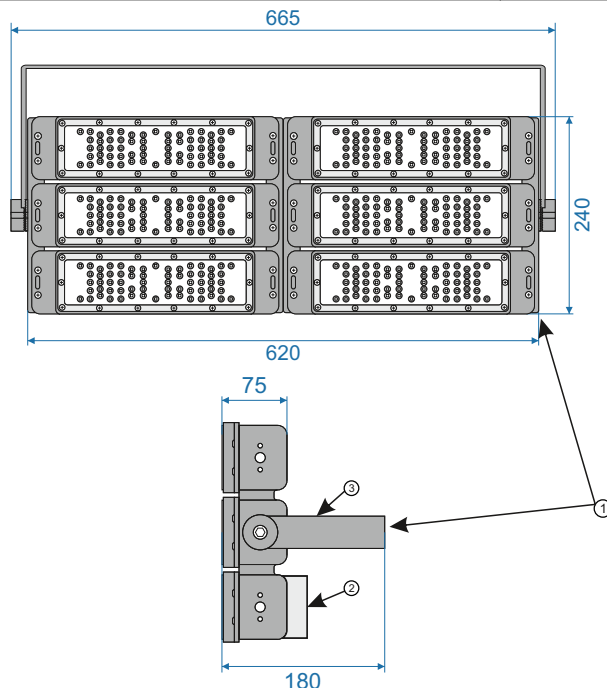
Рисунок 1 — Общий вид изделия
