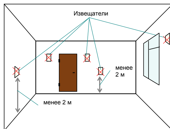
е) НЕрекомендуемые места установки извещателя
