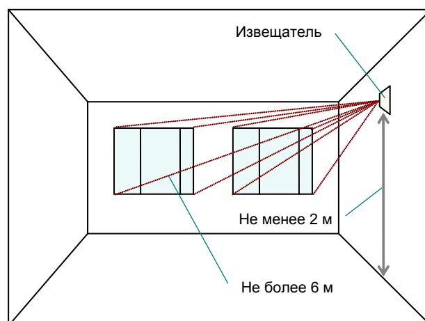
б) установка извещателя на боковой стене
