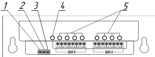
Схема подключения ББП-50 М v8
