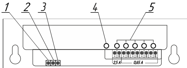
Схема подключения ББП-50 М v5
