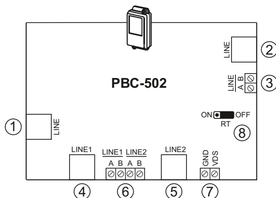
Рисунок 3 - Расположение клемм, разъемов и перемычек разветвителя видеосигнала PBC-502
