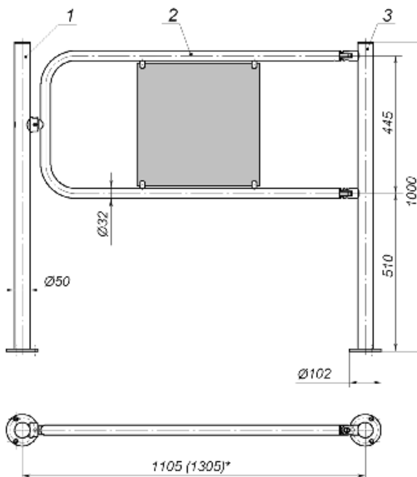
Рисунок 6. Автоматическая поворотная секция ограждения с электромагнитным УБ: 1 – стойка с электромагнитным УБ; 2 – створка; 3 – опорная стойка
