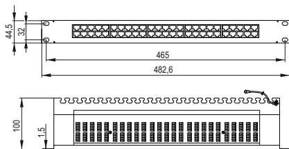
Рисунок/Figure 3 – PP50-1UC03U-D05
