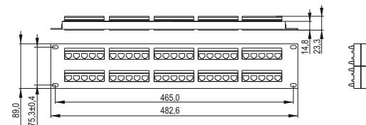
Рисунок/Figure 2 – PP50-2UC03U-110
