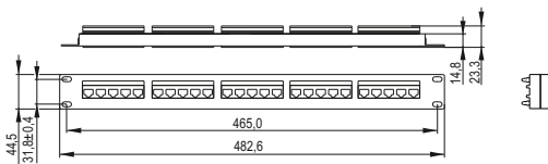
Рисунок/Figure 1 – PP25-1UC03U-110
