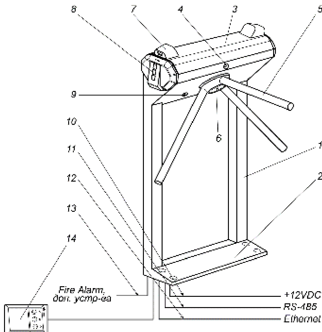
Рисунок 1. Устройство ЭП
