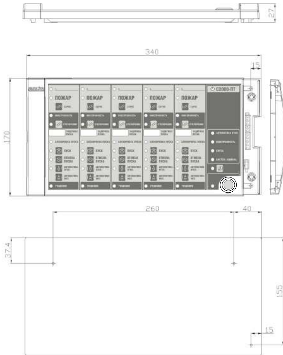
Рисунок 1. Внешний вид, габаритные и установочные размеры блока «C2000-ПТ»
