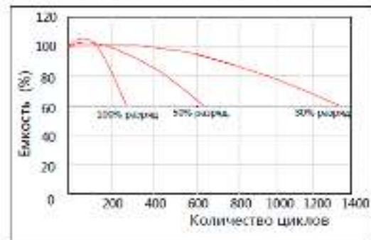
Срок службы в циклическом режиме (25°C)
