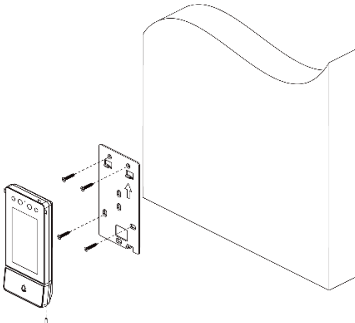
Рисунок 3-3. Накладная установка
