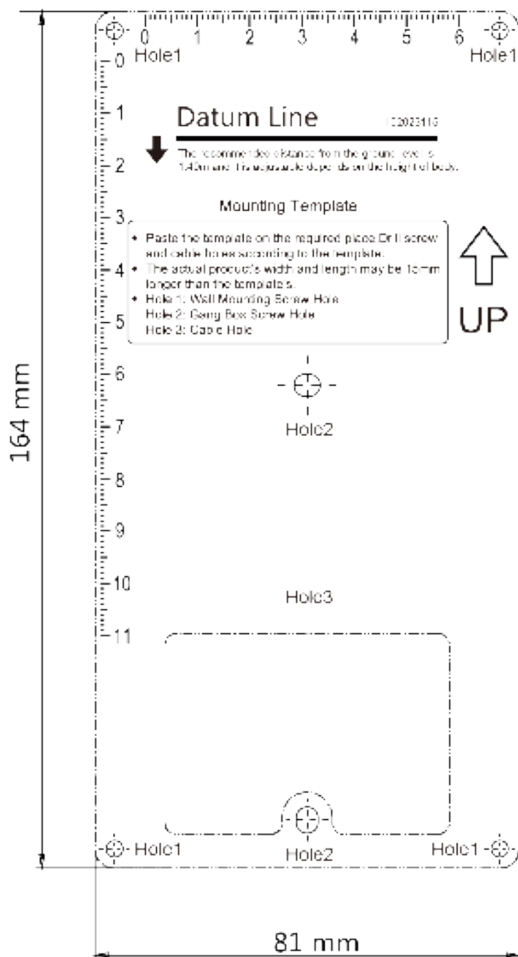
Рисунок 3-2. Монтажный шаблон
