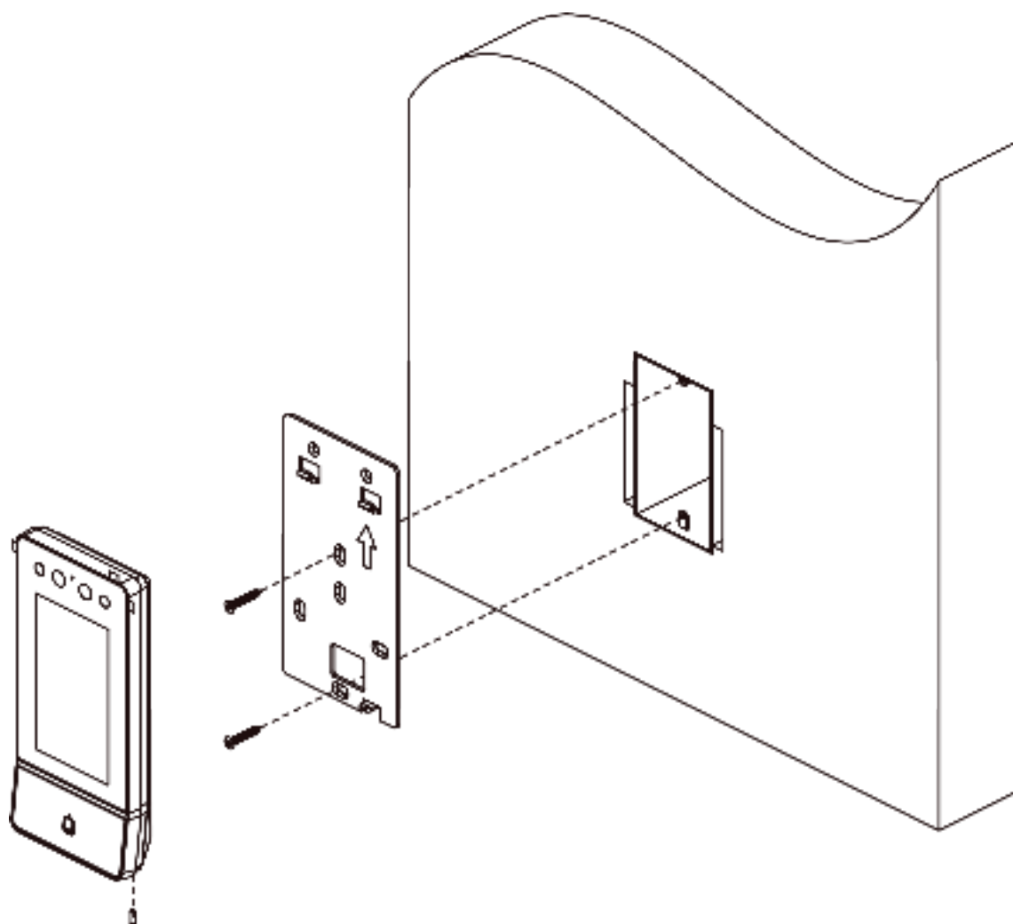
Рисунок 3-4. Врезная установка
