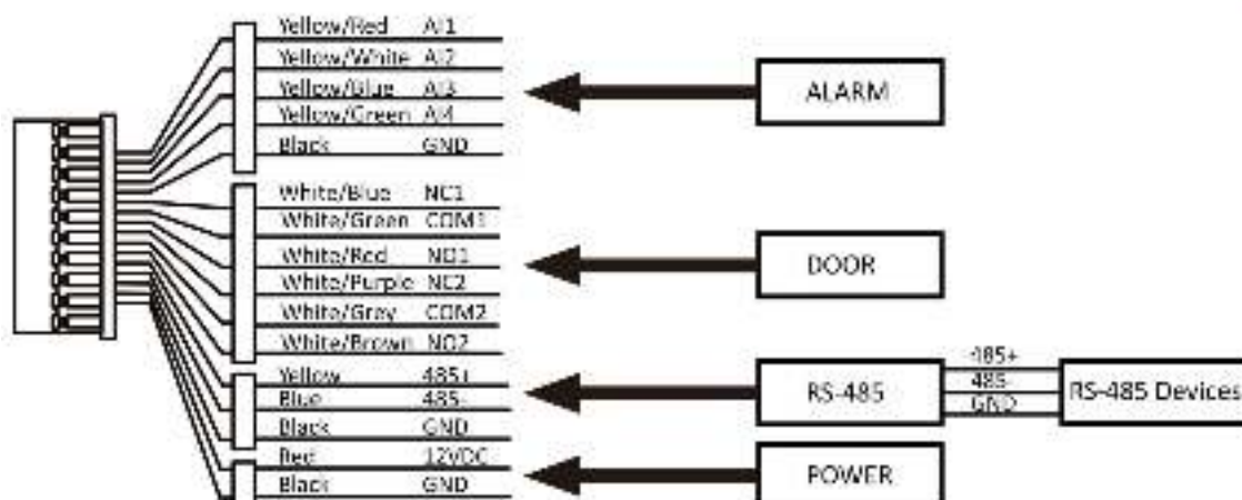
Рисунок 2-1. Описание разъемов
