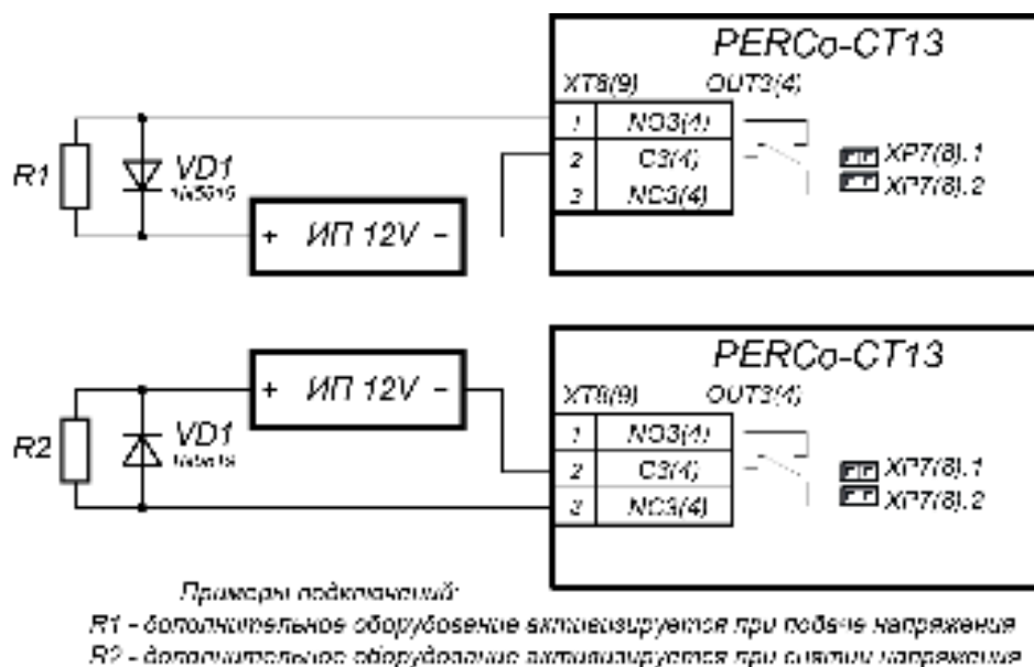
Рисунок 23. Схема подключений дополнительного оборудования к релейным выходам контроллера
