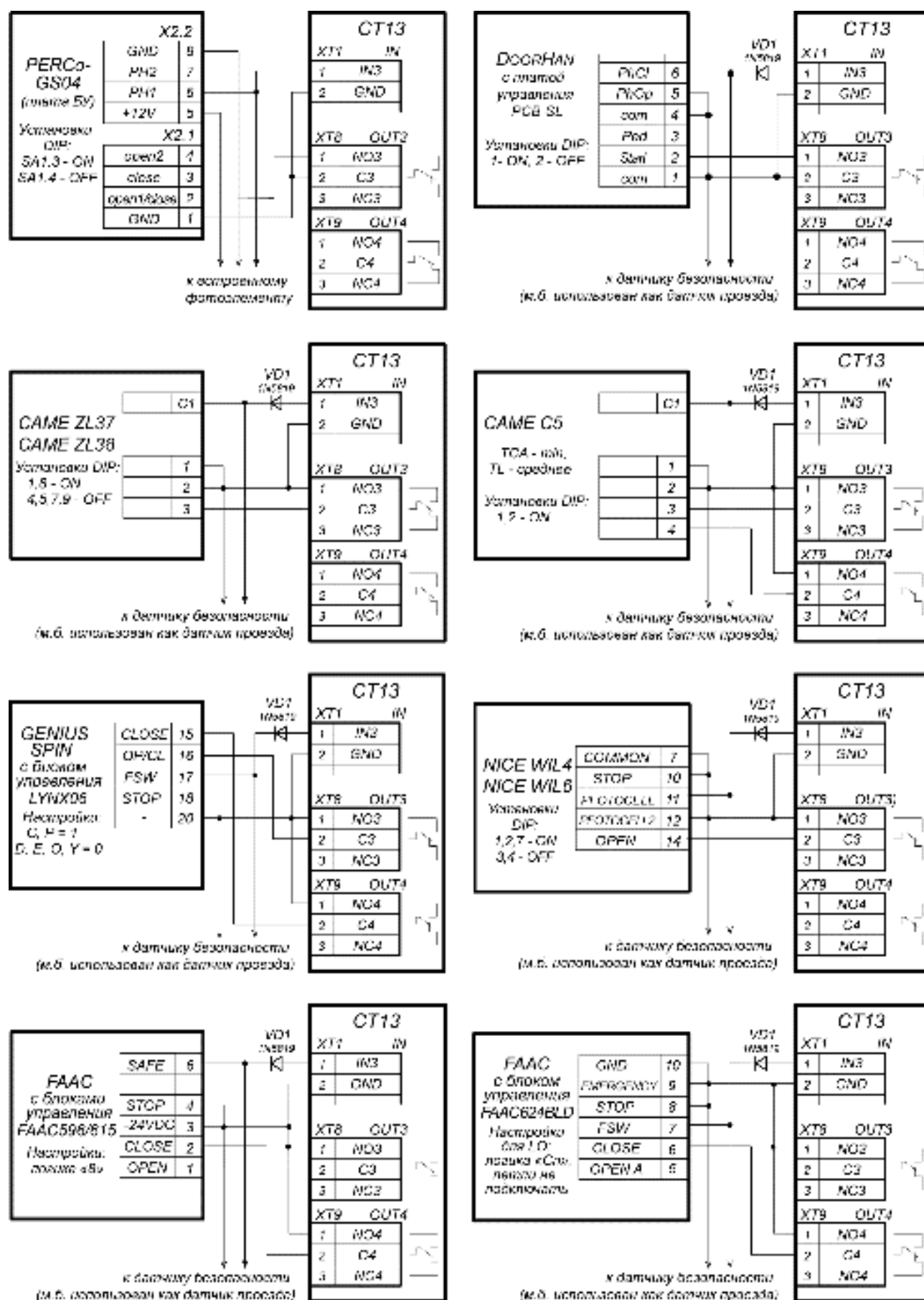
Рисунок 20. Примеры схем подключения шлагбаумов к контроллеру АТП
