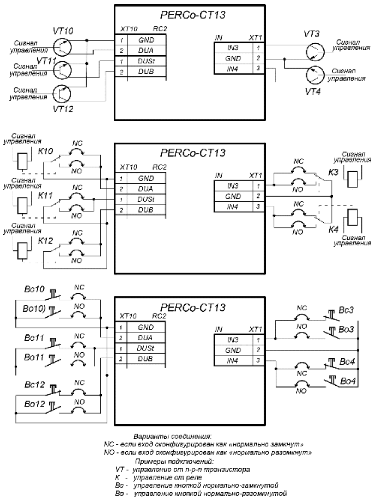
Рисунок 25. Схема подключений доп. оборудования к входам контроллера
