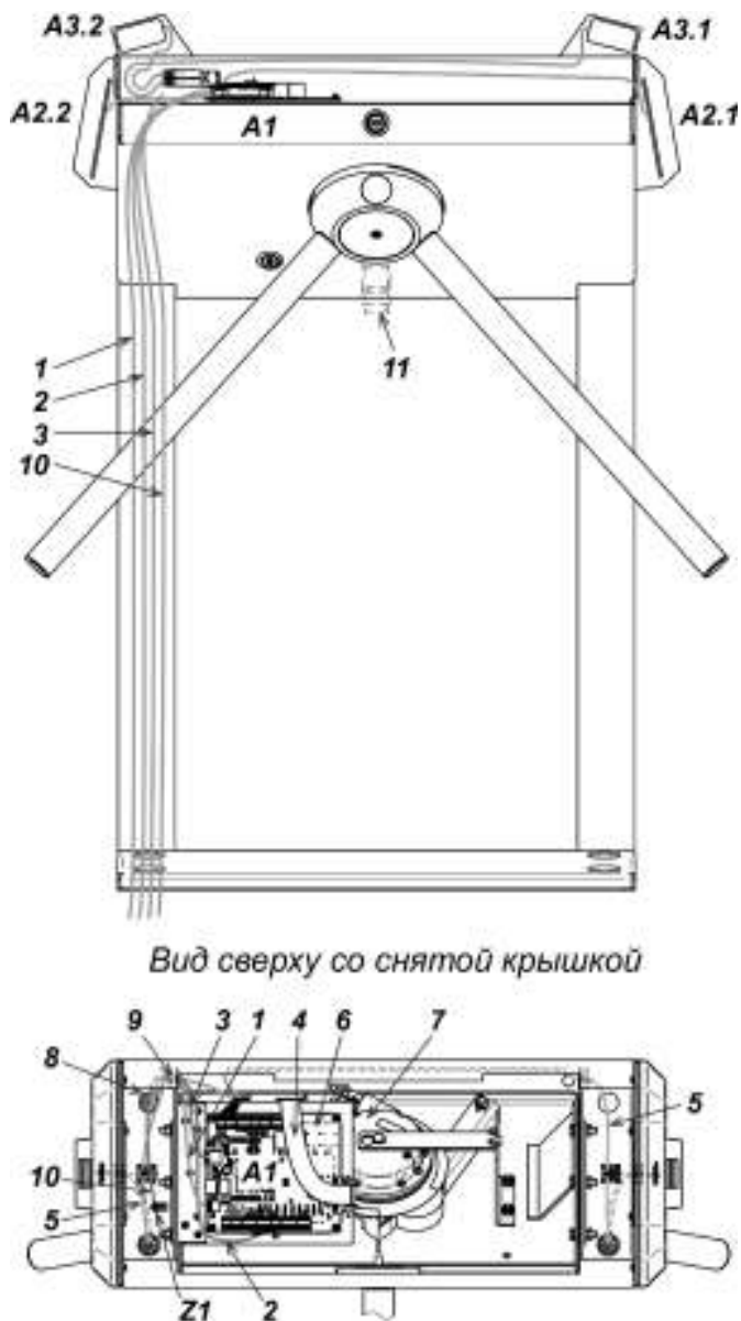
Рисунок 14. Схема прокладки кабелей в стойке ЭП
