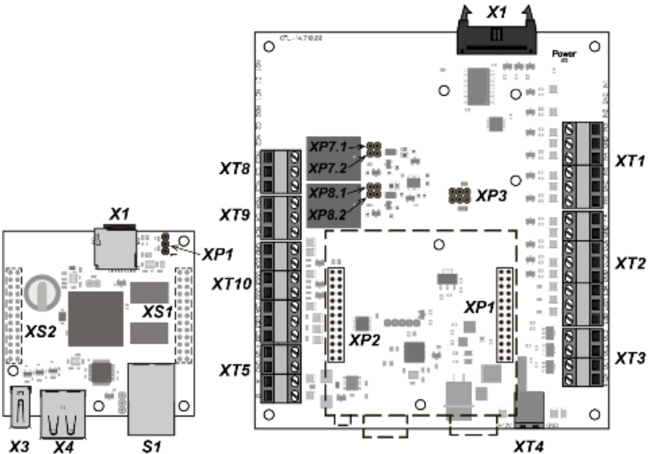
Рисунок 8. Внешний вид верхней и нижней плат контроллера Таблица 2. Назначение разъемов контроллера (см. рис. 8)
