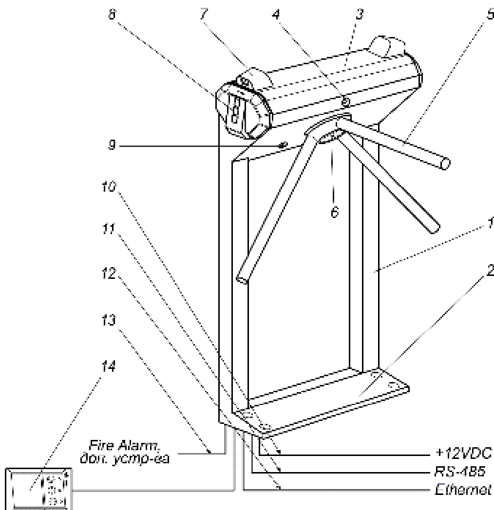
Рисунок 2. Устройство ЭП
