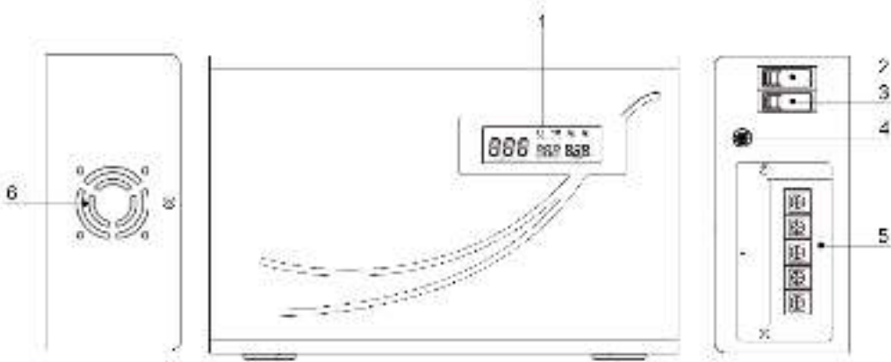
Рисунок 3. Внешний вид стабилизаторов напряжения SMARTWATT AVR TRIAC 3000-10000VA. Описание элементов приводится в таблице 3.
