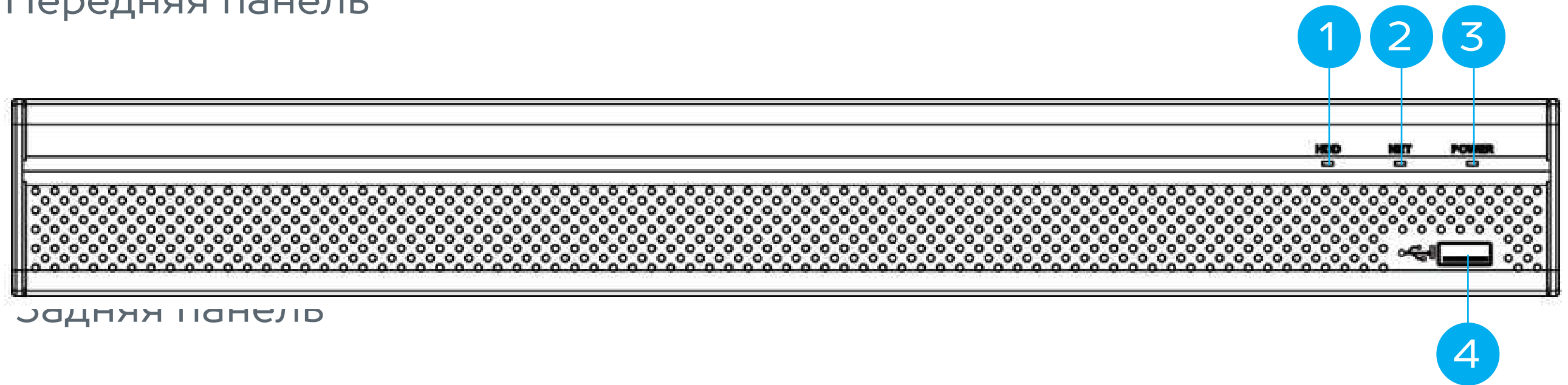
Передняя панель
