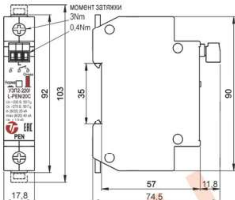
Рис.1 Габаритные размеры
