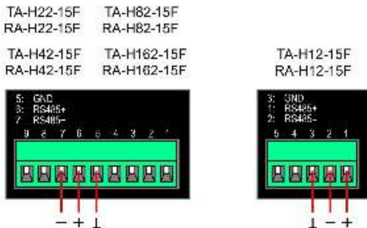
Рис.12 Клеммные колодки для подключения устройств с интерфейсами RS485 к передатчикам / приемникам TA-Hxx-15F / RA-Hxx-15F
