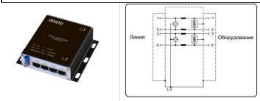
Рис.4 Внешний вид и электрическая схема SP-IP4/100
