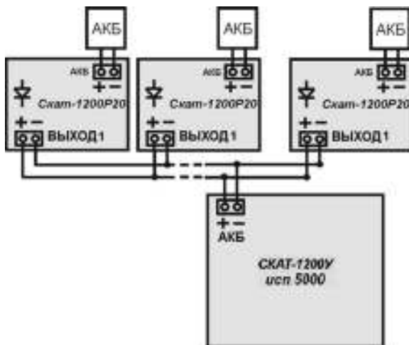
Рисунок 5. Схема каскадного подключения изделия.
