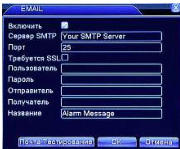
Рис. 4.20 EMAIL
