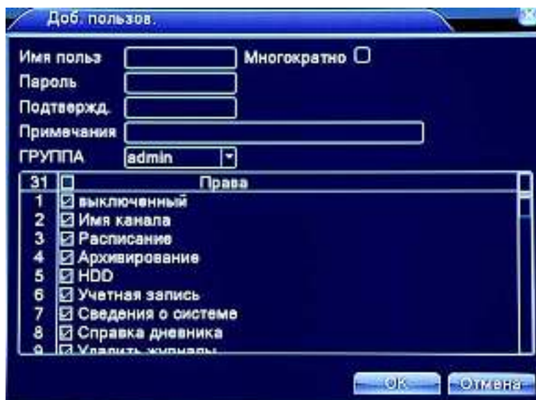
Рис 4.35 Добавление пользователя
