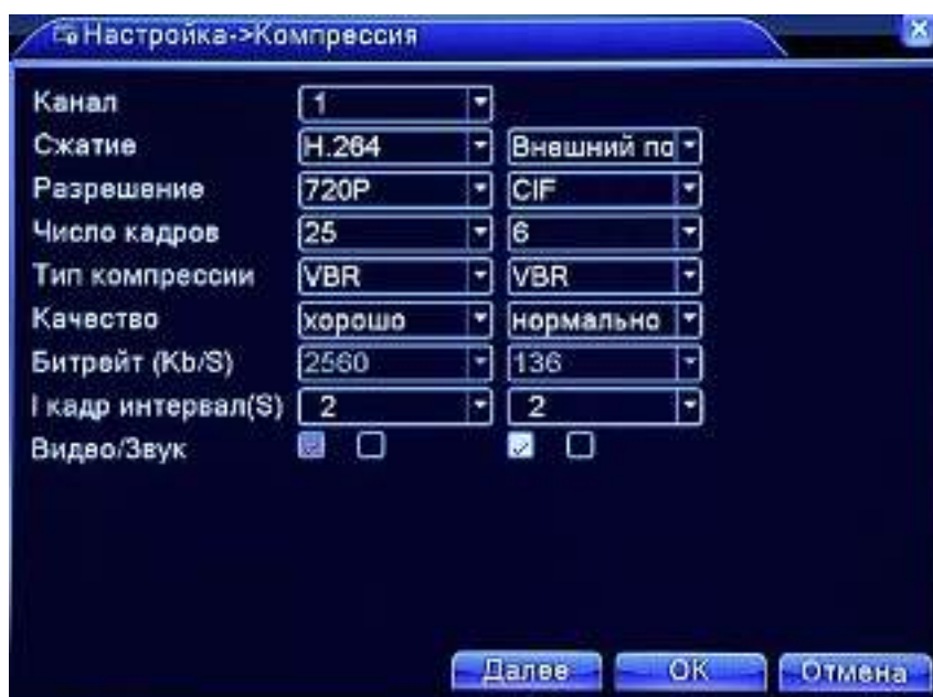
Рис. 4.15 Настройки кодирования
