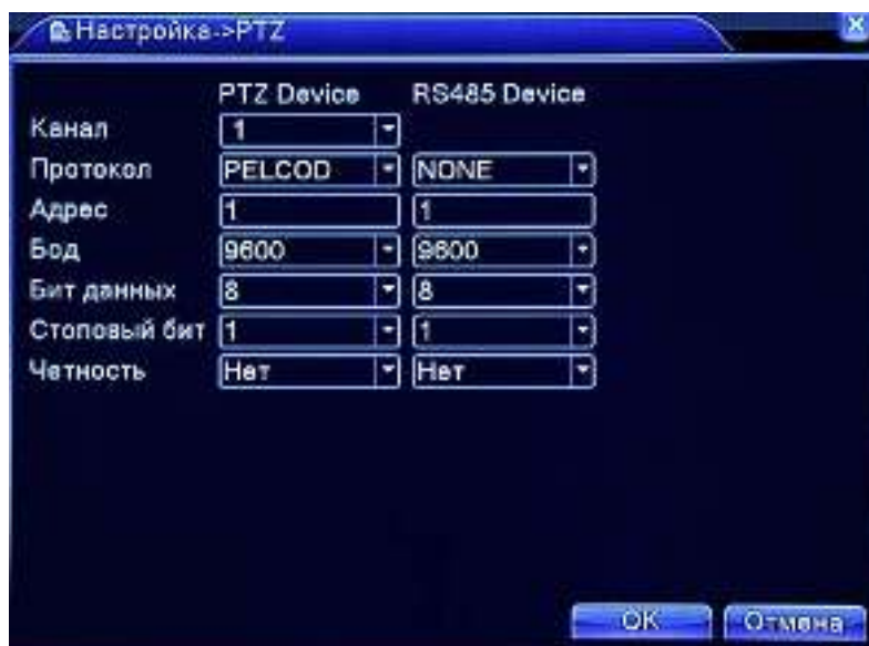
Рис. 4.31 Настройка PTZ
