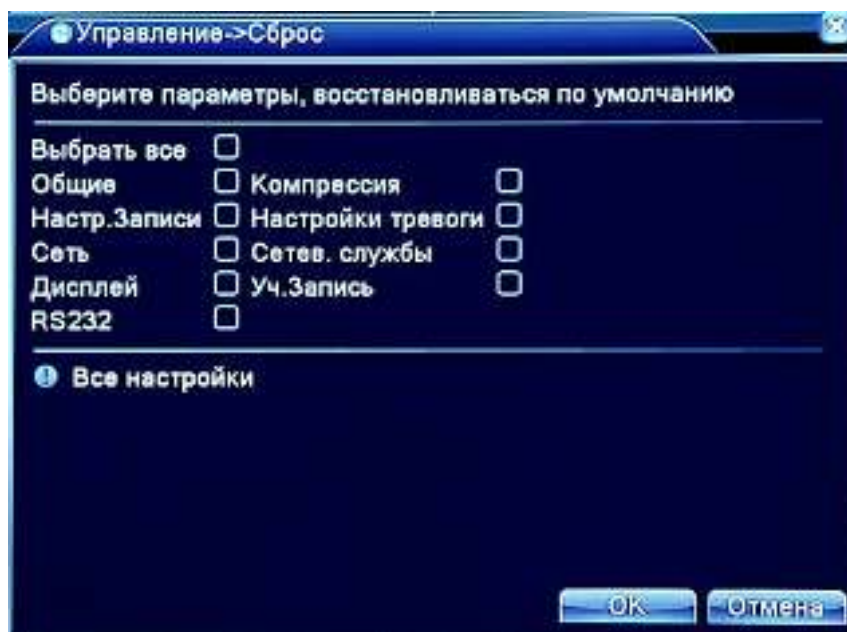
Рис 4.40 Восстановление
