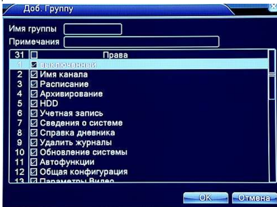
Рис 4.36 Добавление группы
