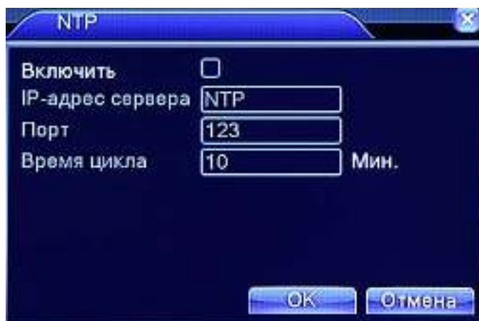
Рис. 4.19 NTP сервер
