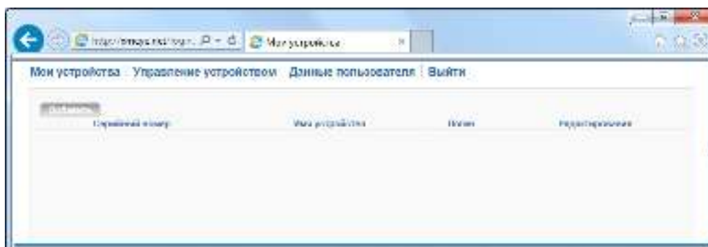
Рис. 5.4 Добавление устройства
