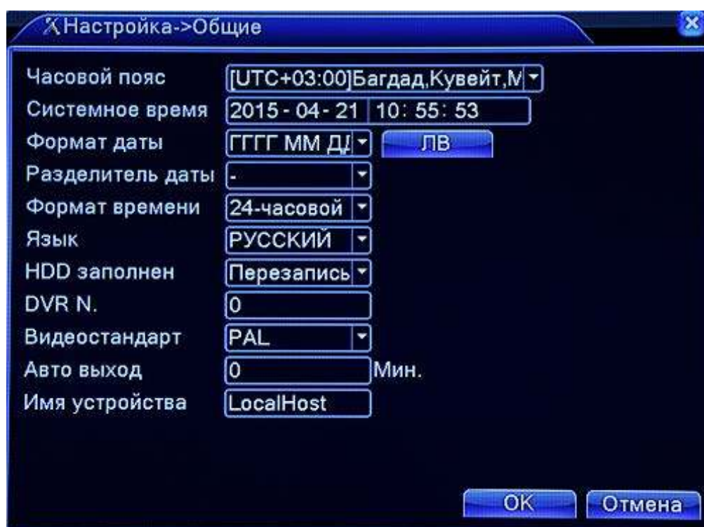
Рис. 4.12 Общие настройки
