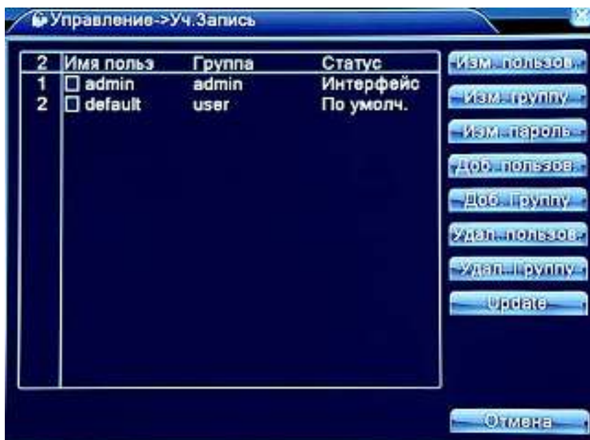
Рис. 4.33 Учетные записи
