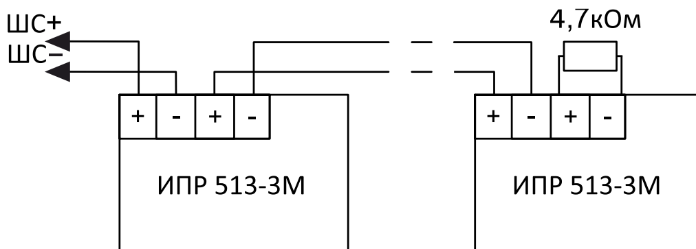
Рисунок 2.3. Схемы подключения извещателей в ШС прибора (продолжение)
