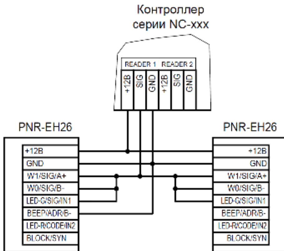
Рисунок 10. Подключение двух считывателей в режиме Parsec одним кабелем
