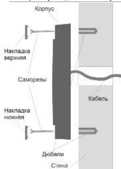
Рисунок 2. Крепление считывателя
