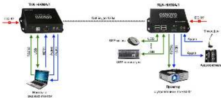
Рис.4 Типовая схема подключения комплекта TLN-HiKMA/1+RLN-HiKMA/1
