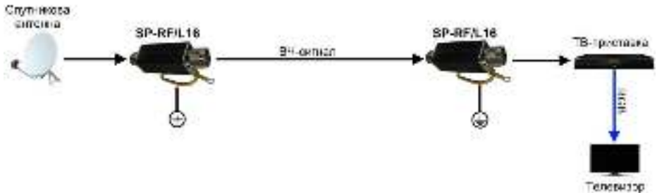
Рис.3 Схема подключения устройств грозозащиты SP-RF/L16
