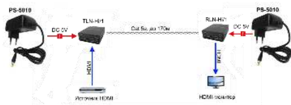
Рис.2 Типовая схема подключения блока питания PS-5010
