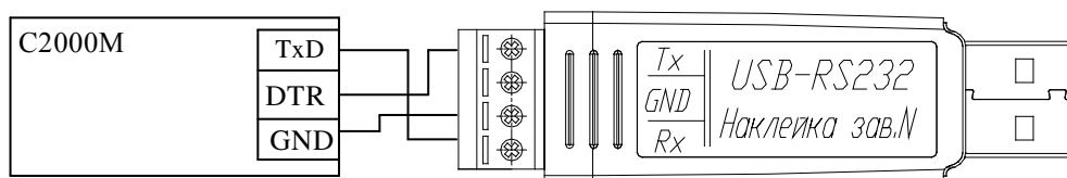
Рис.2.2 Схема подключения «USB-RS232» к пульту «C2000M»
