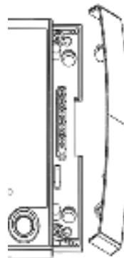
Рисунок 2. Снятие боковой крышки
