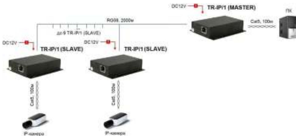
Рис. 4 Схема подключения TR-IP/1(MASTER) и TR-IP/1(SLAVE) для организации системы IP-видеонаблюдения.
