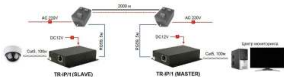
Рис. 7 Схема подключения TR-IP/1(MASTER) и TR-IP/1(SLAVE) для передачи данных по силовым линиям питания AC 220V.
