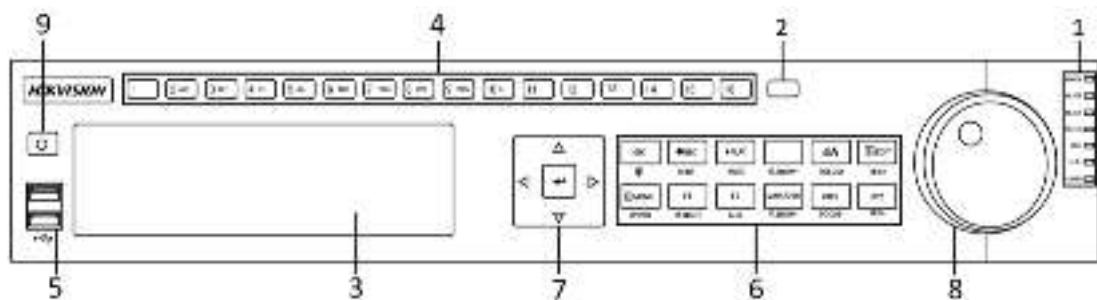
Рисунок 1-3 Серия DS-8600NI-I8
