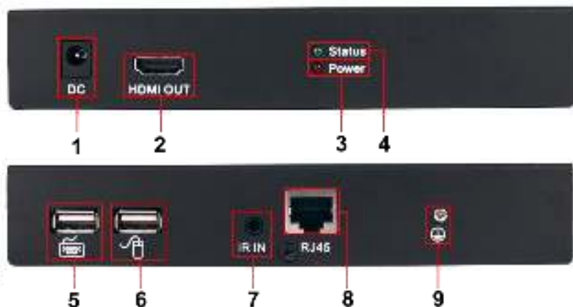
Рис. 4 Приемник RLN-HiKM/1(ver.2), разъемы и индикаторы передней и задней панели
