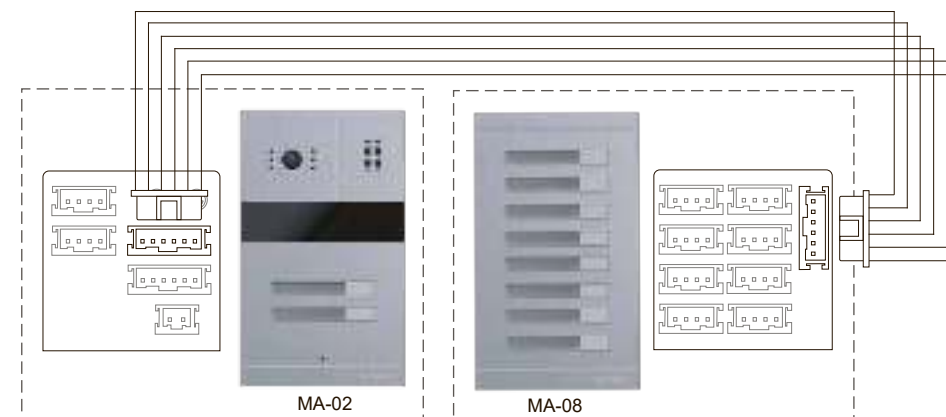
Схема 4. Подключение MA-02 и MA-08.
