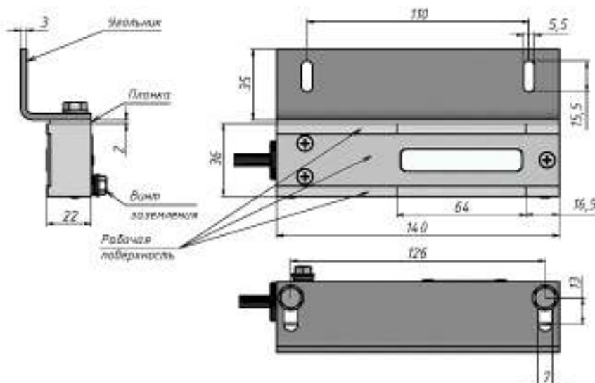
Рисунок 4 - Корпусная часть
