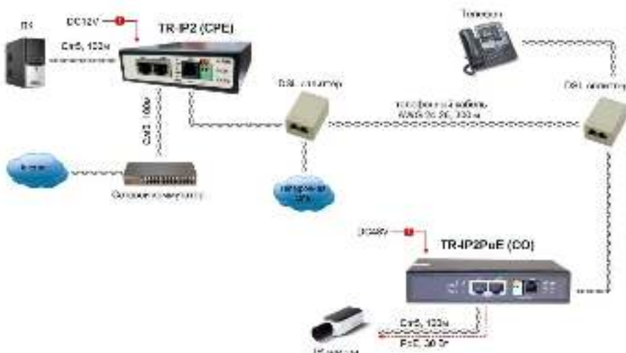
Рис. 7б Схема подключения TR-IP2PoE (CO) и TR-IP2 (CPE) для организации IP-видеонаблюдения с параллельным подключением телефонного аппарата
