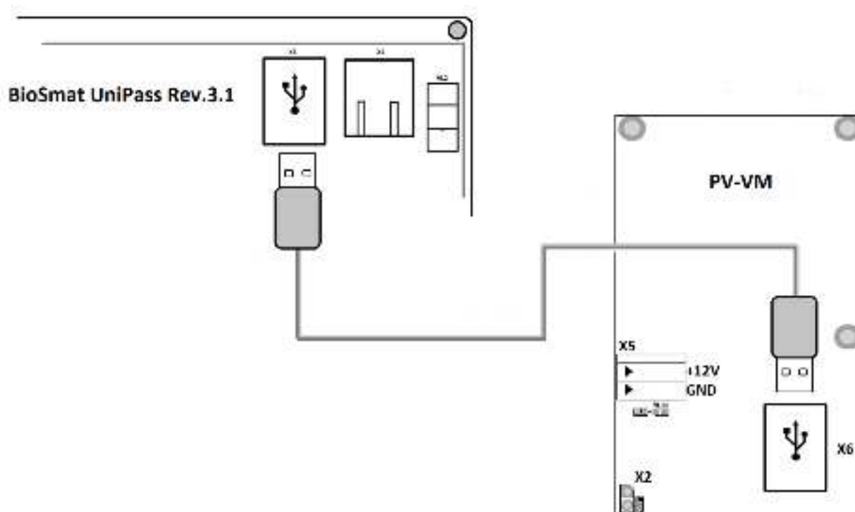
Рисунок 7. Схема подключения к контроллеру BioSmart UniPass
