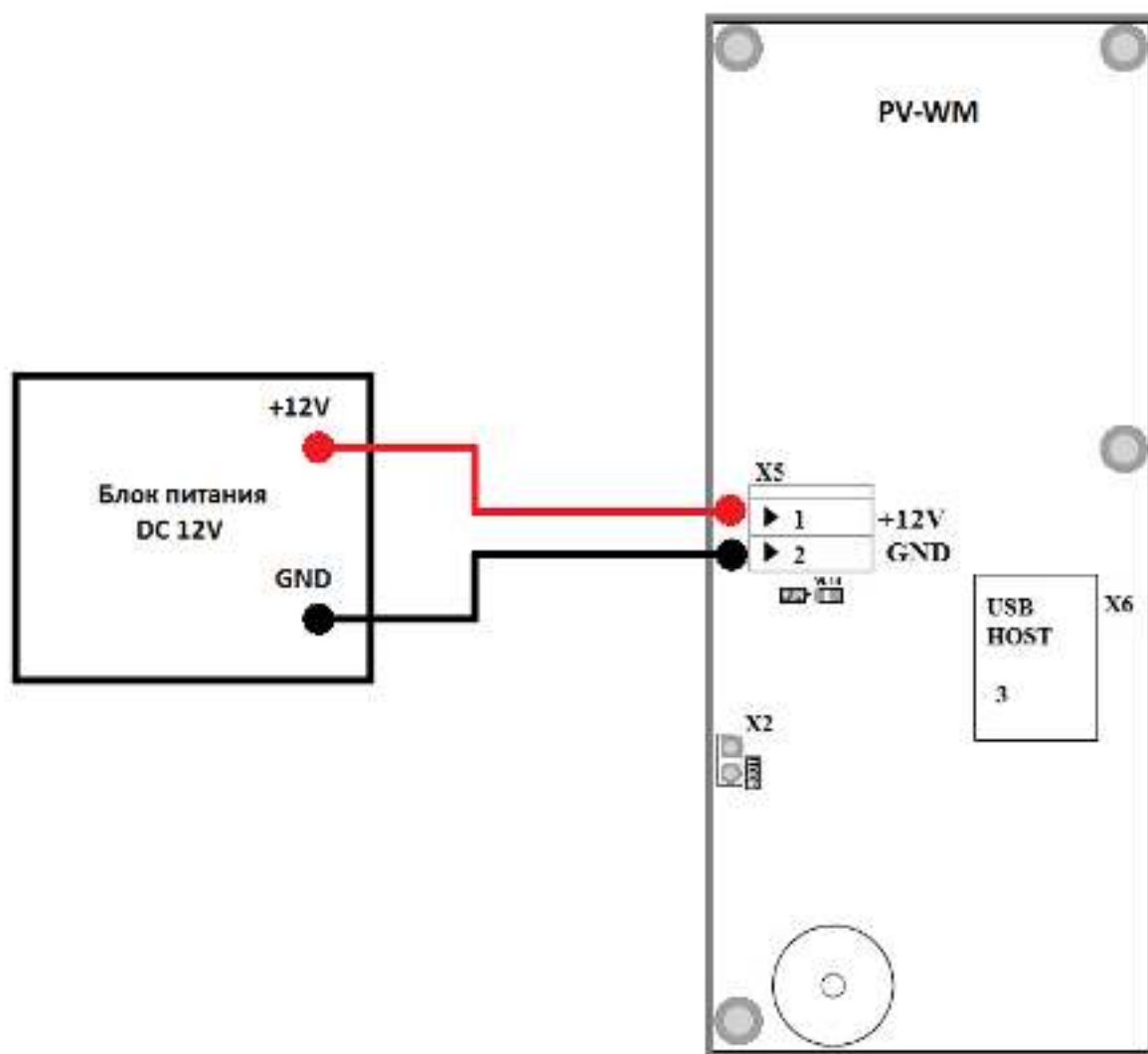
Рисунок 6. Схема подключения питания считывателя
