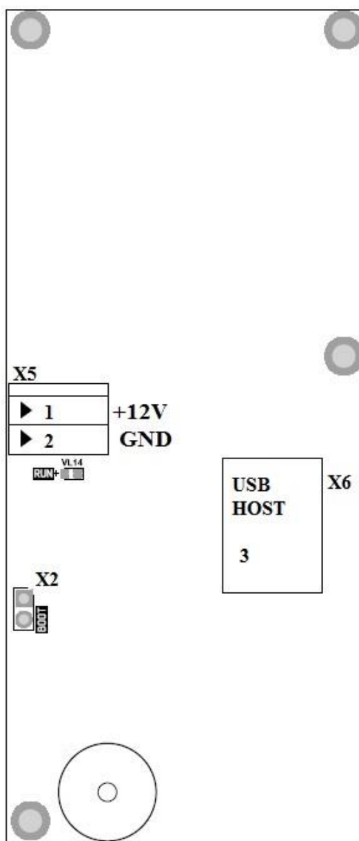
Рисунок 2. Внешний вид печатной платы считывателя
