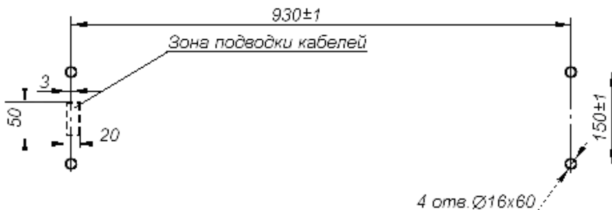
Рисунок 11. Схема разметки отверстий для крепления стойки турникета
