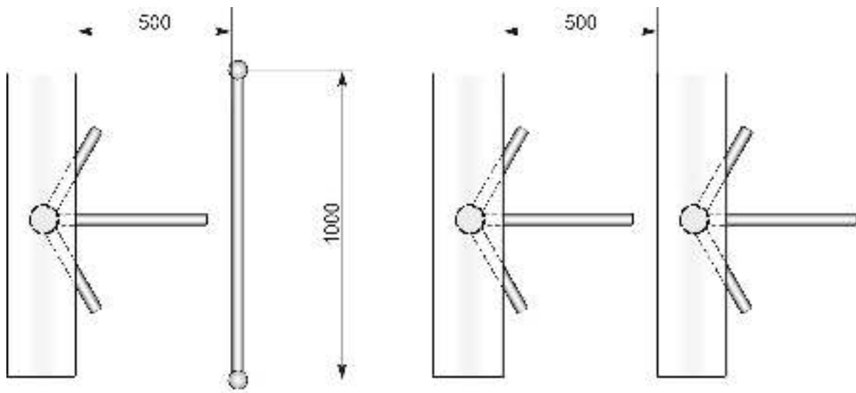
Рисунок 10. Рекомендации по организации зоны прохода
