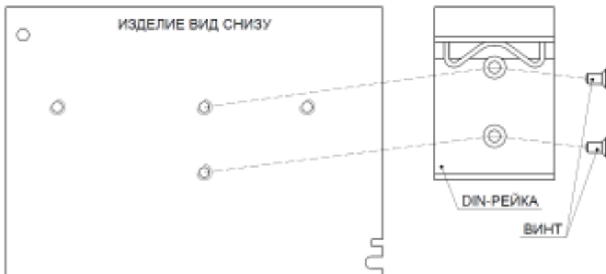
Рисунок 2 – крепление DIN-рейки.
