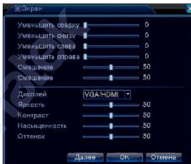
Рис. 3.20 Настройка ТВ выхода
