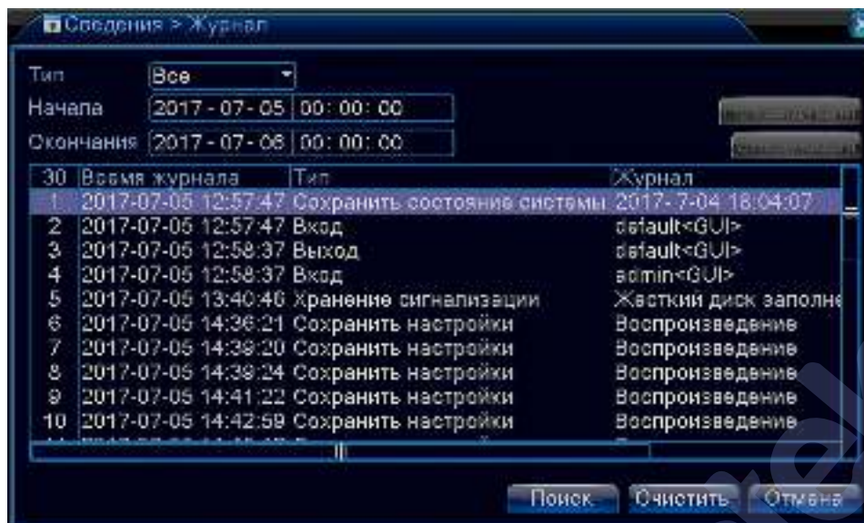
Рис 4.63 Журнал системных событий.
