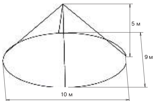
Рисунок 1 – Вид зоны обнаружения ИК канала
