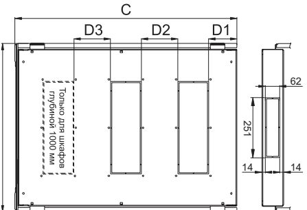
ВИД СНИЗУ
