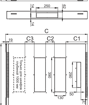
ВИД СВЕРХУ
