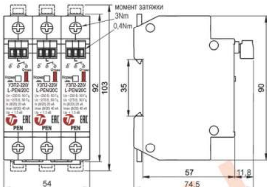
Рис.1 Габаритные размеры
