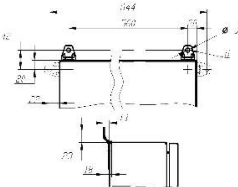
Рисунок 4 – Пример установки кронштейнов
