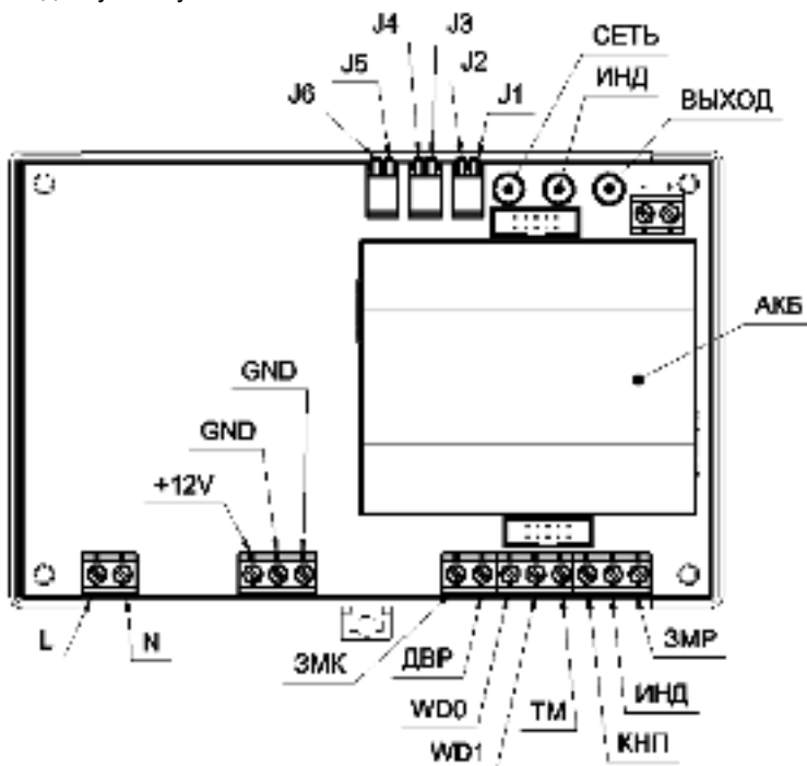
Рисунок 1 – Элементы подключения.
