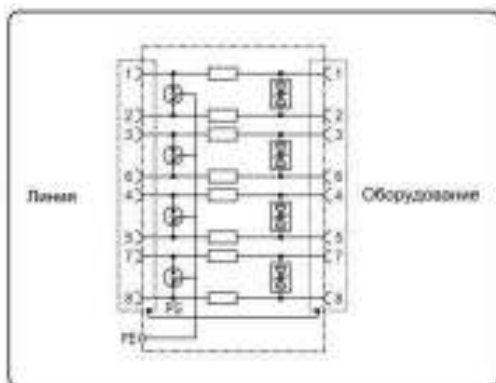
Рис.1 Внешний вид и электрическая схема SP-IP/1000(ver.2), SP-IP/1000D
