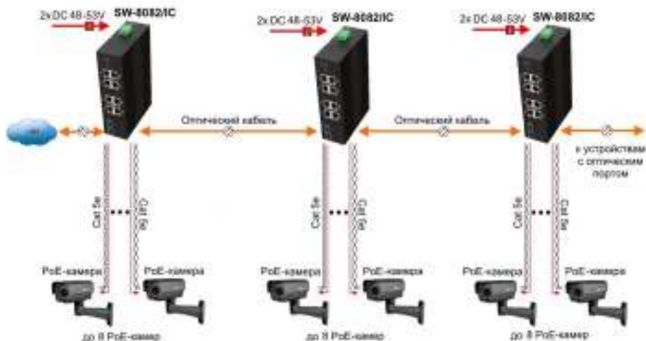
Рис.4 Типовая схема подключения коммутатора SW-8082/IC
