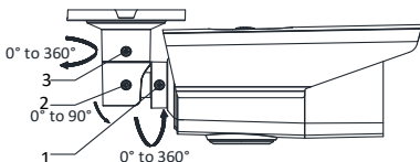
Рисунок 2-3 3-х осевая установка
