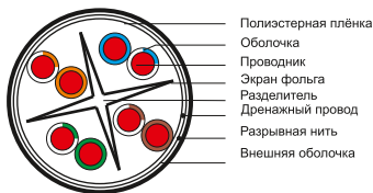
Рисунок 3 – Конструкция кабеля типа F/UTP
