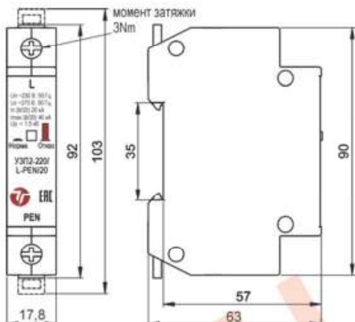
Рис.1 Габаритные размеры
