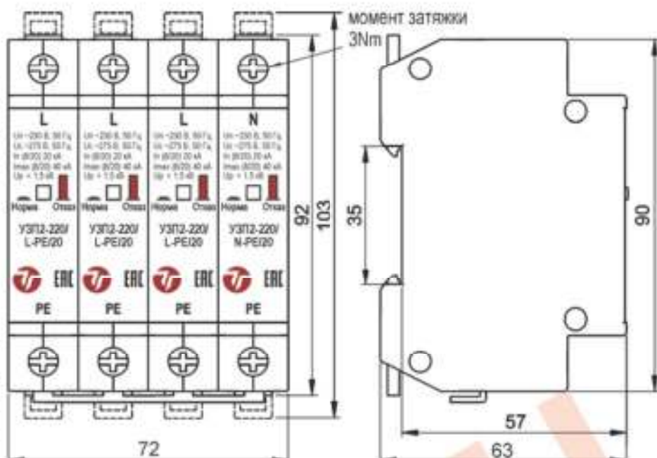
Рис.1 Габаритные размеры
