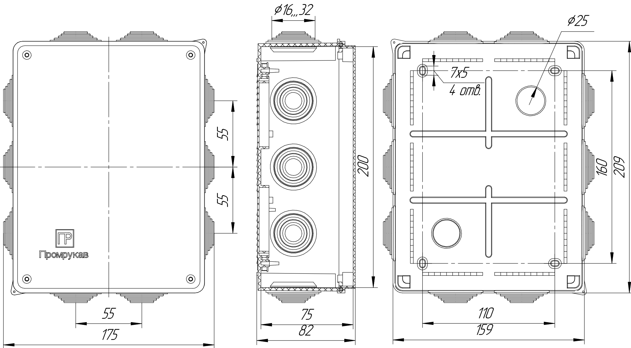
Коробка распределительная 40-0325 для о/п безгалогенная (HF) атмосферостойкая 200x150x75
