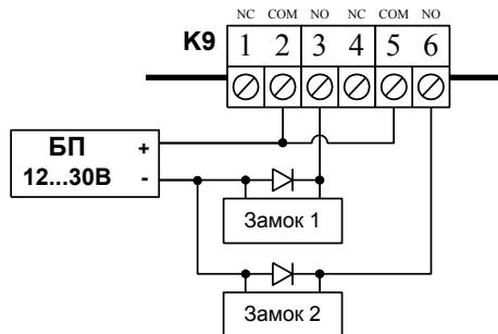
Пример 4. Подключение электромеханического замка (двухдверный и шлюзового режимы)
